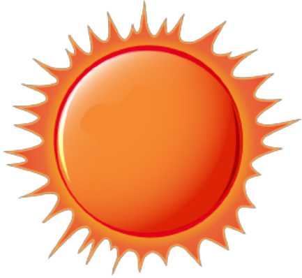
Solen
